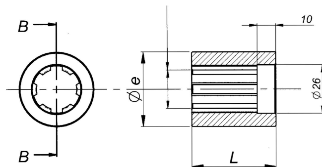
SEZ.: B-B
